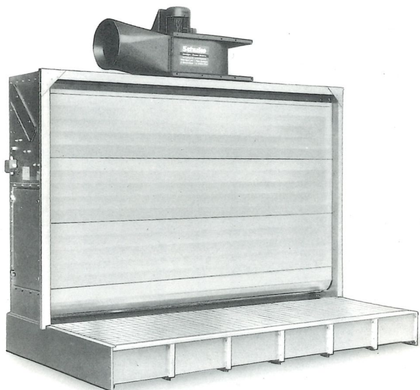
Wasserberieselte Farbnebel-Absaugwand Typ FAW
