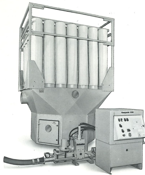
Brikettierpresse Baureihe „Compacto“
