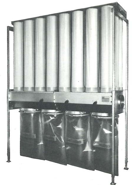
Absackanlage für Späne Baureihe Spa 230
